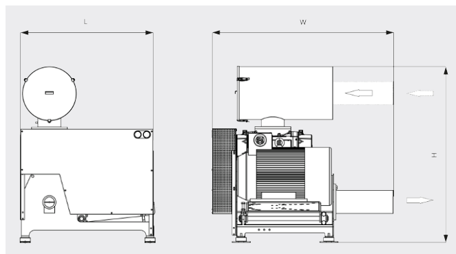
尺寸图 (不含隔音罩)
