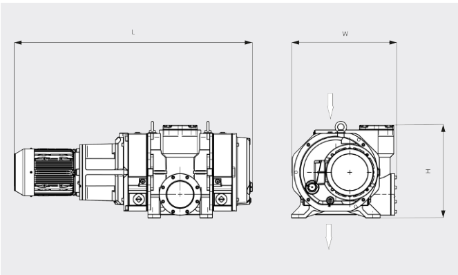
尺寸图
