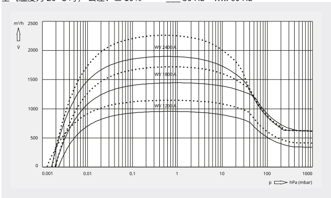
抽气速率
