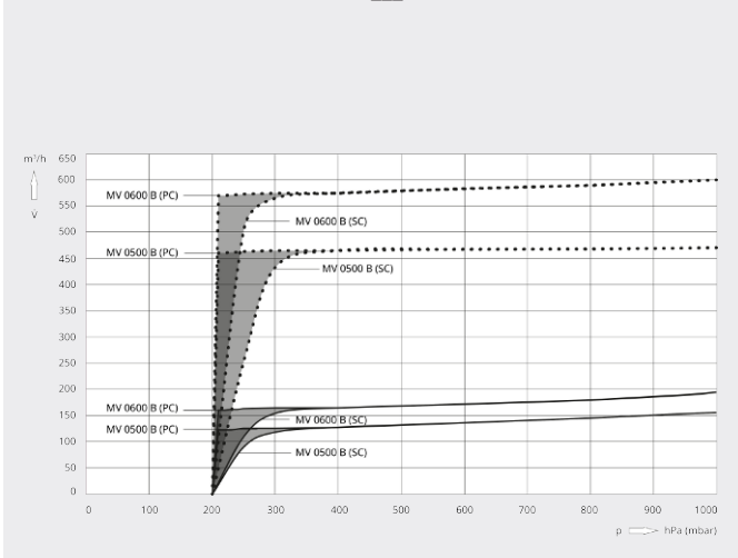
抽气速率
